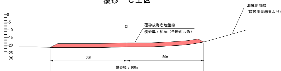
覆砂 C 工区
