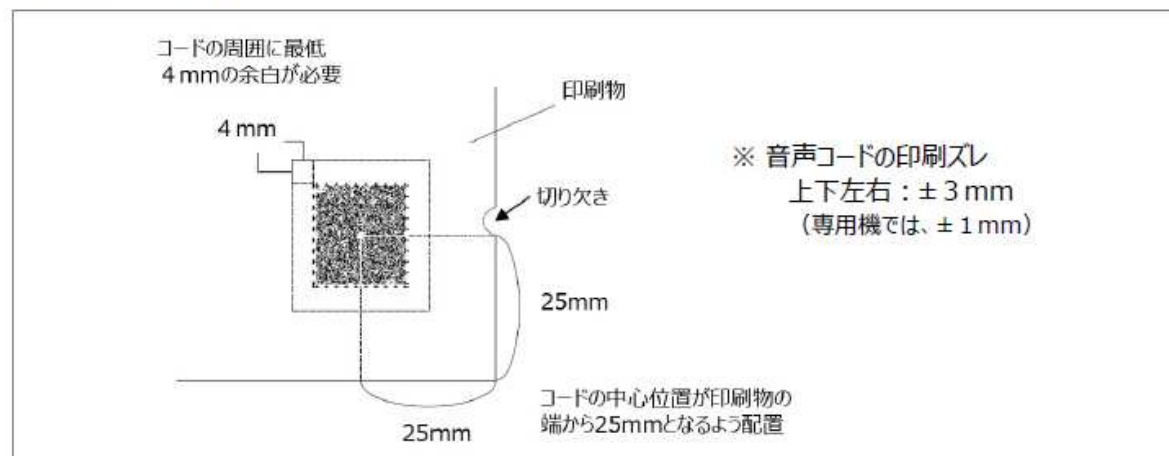
(図) 音声コードの印刷位置
