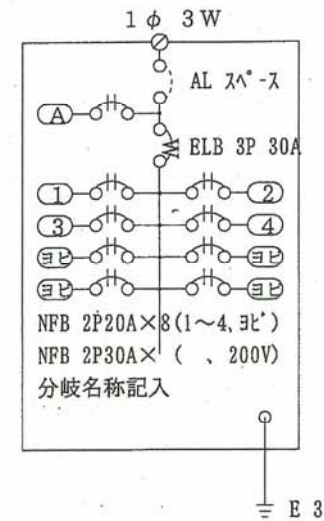
分電盤 L-1
