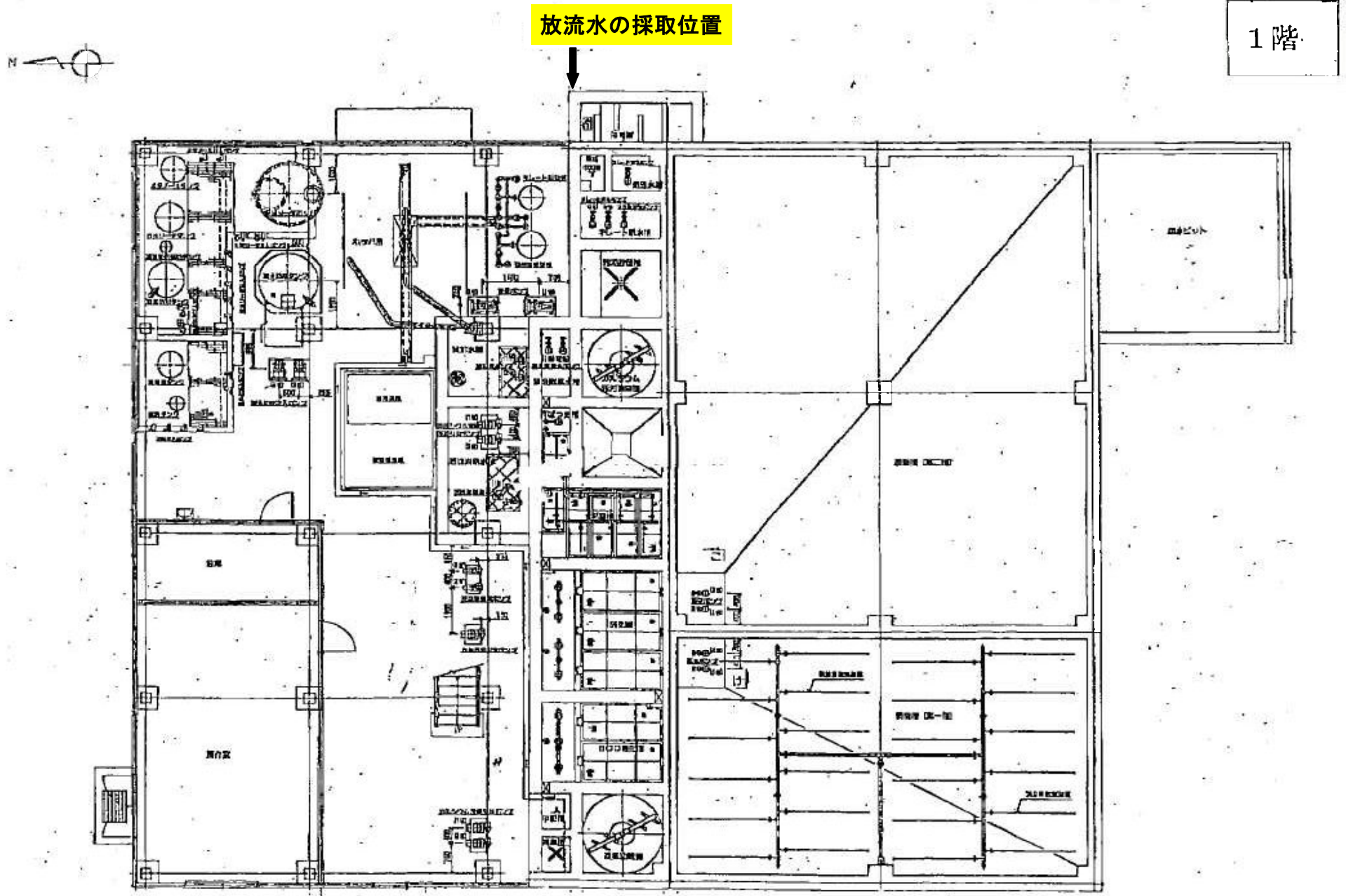
(図2) 蒲江一般廃棄物最終処分場 放流水の測定箇所を記した配置図
